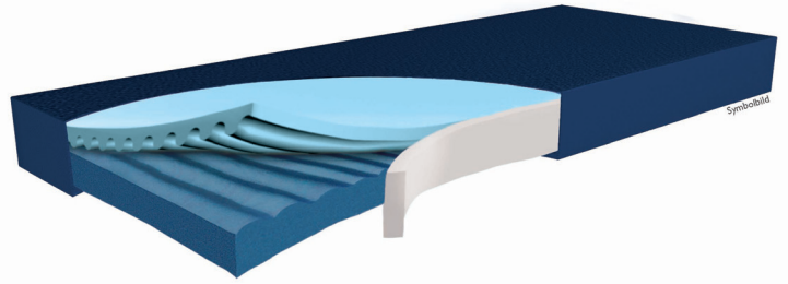
Abb. Matratzenquerschnitt
